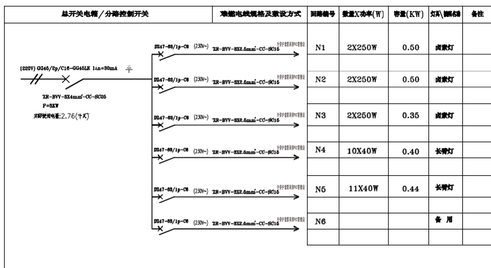
配电系统图
