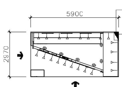
电气平面图 1:100
